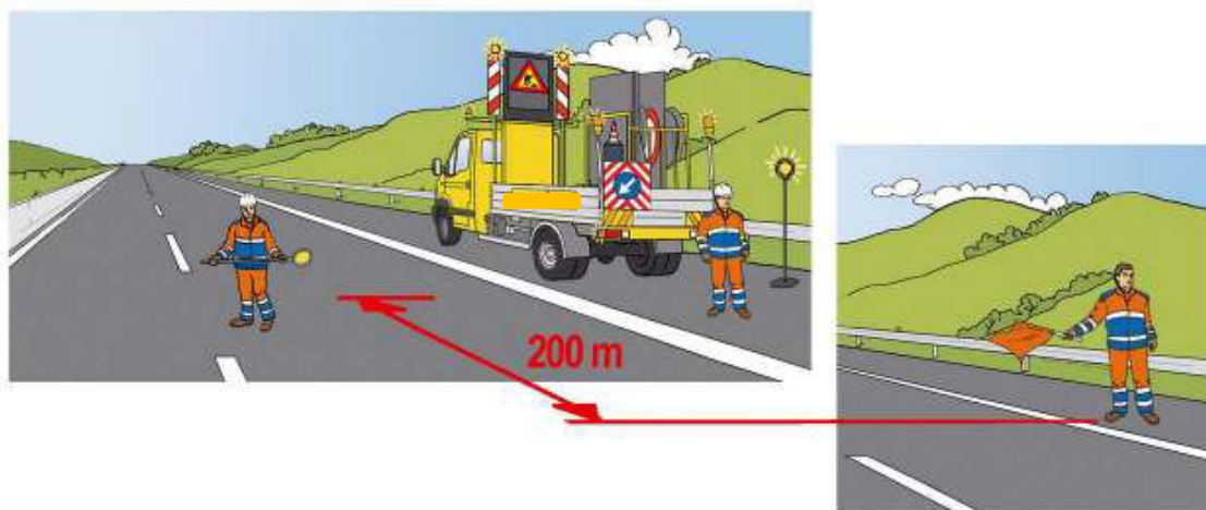
Figura 24 – Chiusura della corsia di marcia: installazione delle lampade blitz
