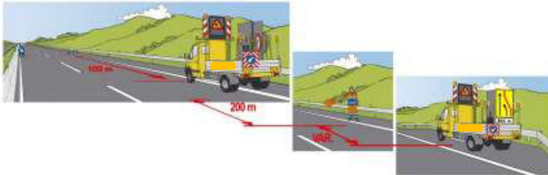
Figura 54 – Chiusura della corsia di sorpasso: installazione della segnaletica di testata sul margine sinistro
