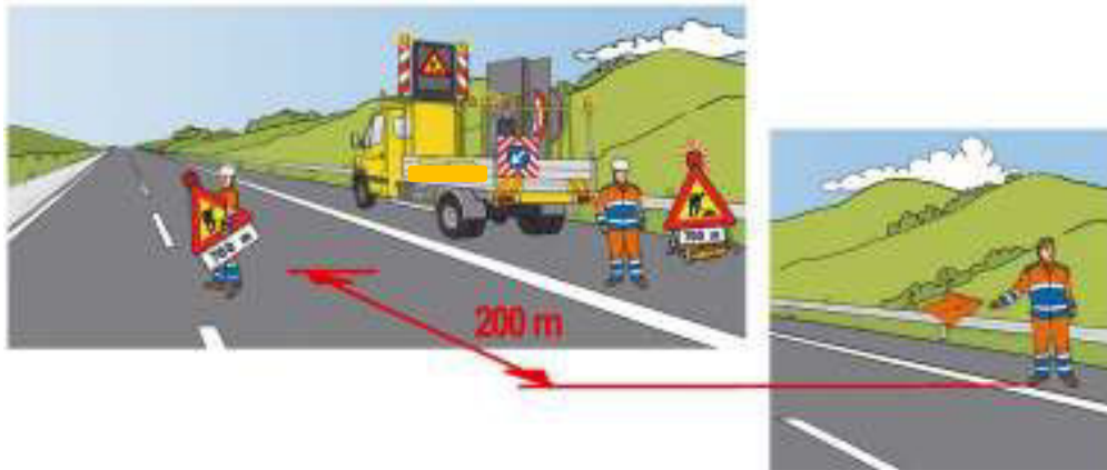
Figura 35 – Chiusura della corsia di sorpasso: installazione del segnale lavori sul margine sinistro
