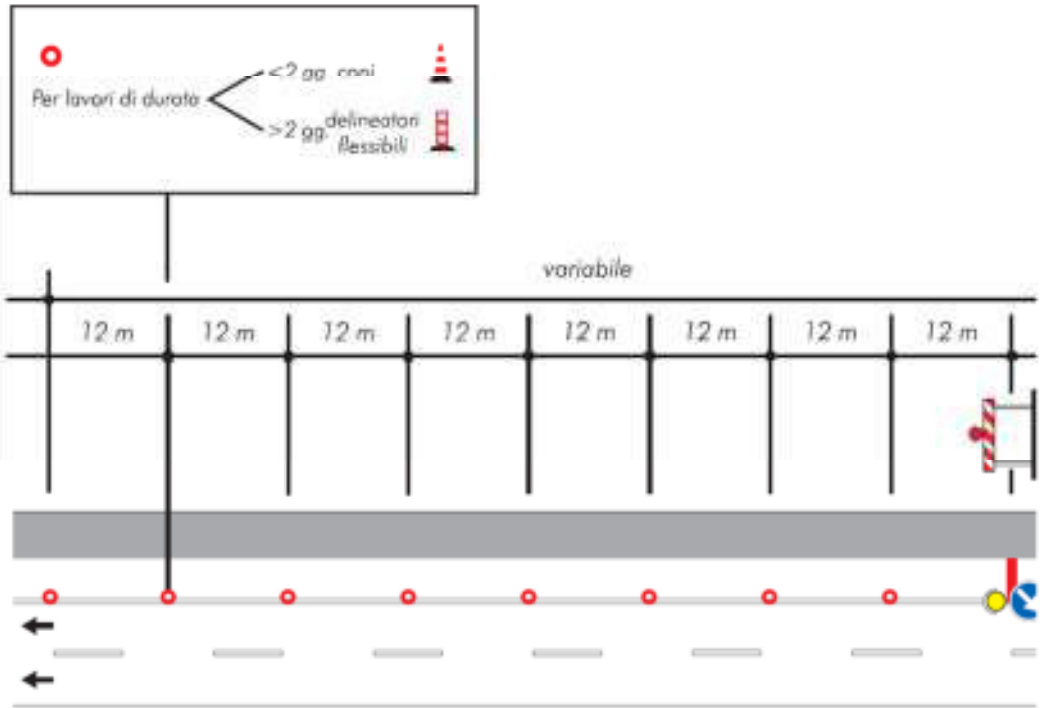
fig. 7 Segnaletica di posizione – delimitazione longitudinale dell'area interessata dal cantiere realizzata con coni o delineatori flessibili
