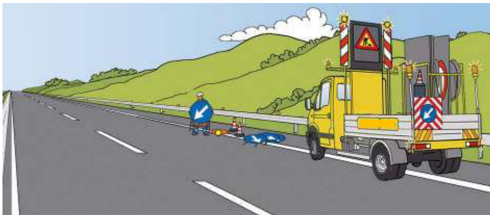
Figura 47 – Chiusura della corsia di marcia: scarico della segnaletica di testata sul margine destro
