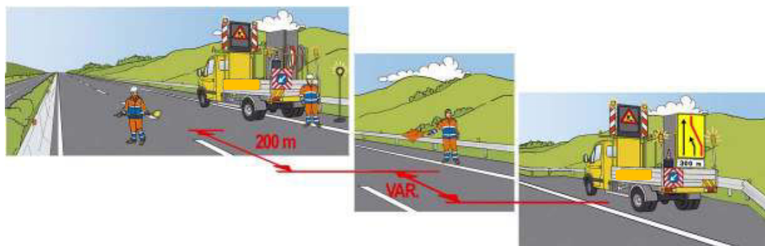
Figura 50 – Chiusura della corsia di sorpasso: installazione della lampada blitz sul margine sinistro
