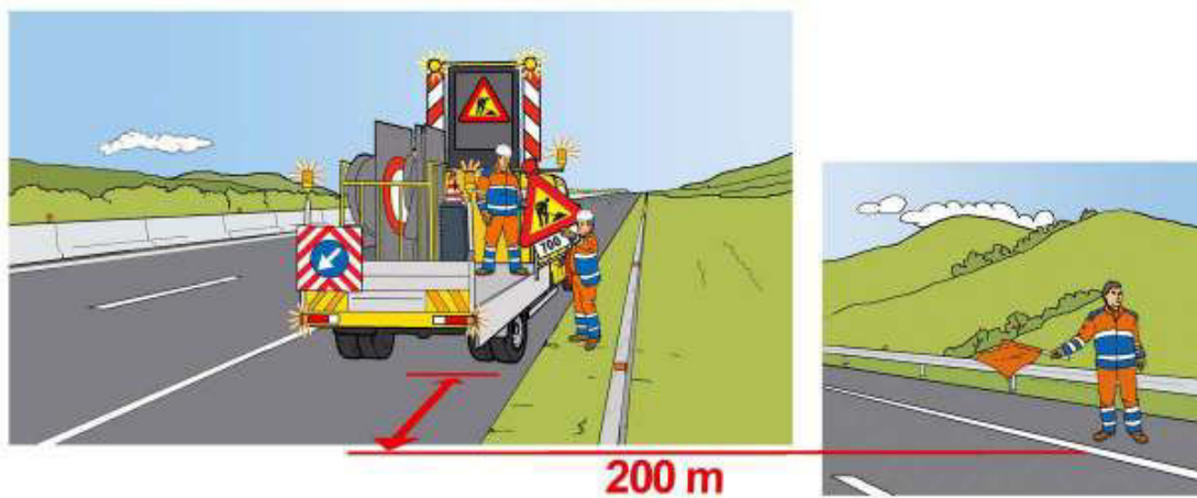
Figura 25 – Chiusura della corsia di marcia: scarico ed installazione del segnale lavori sul margine destroy
