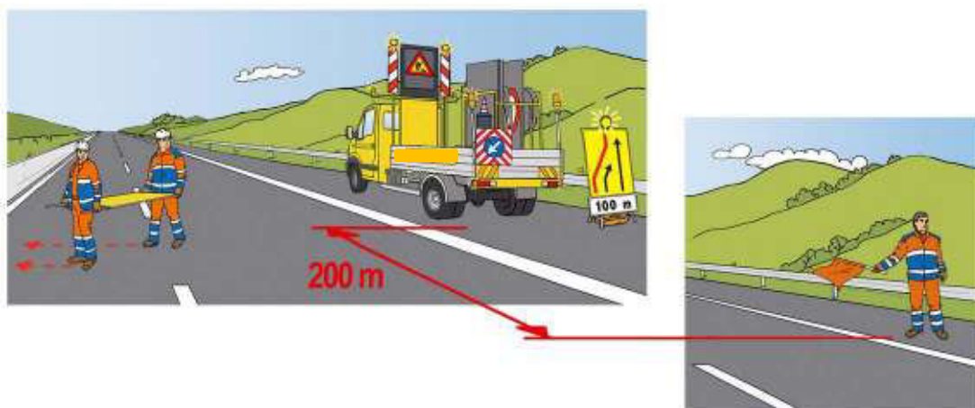
Figura 37 – Chiusura della corsia di sorpasso: trasporto del segnale di esclusione della corsia sul margine sinistro
