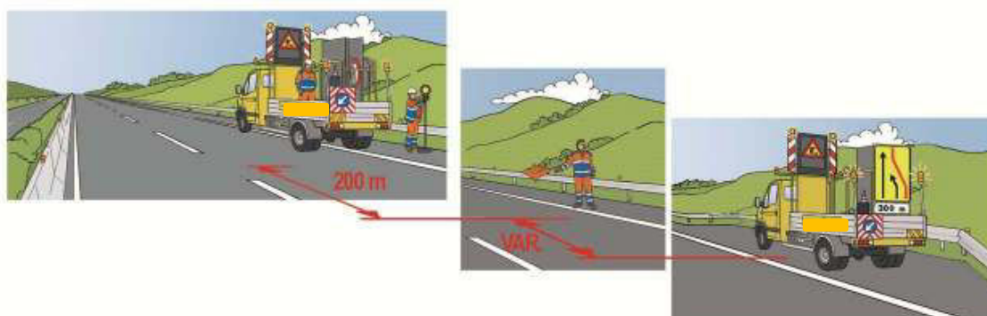
Figura 49 - Chiusura della corsia di sorpasso: configurazione mezzo di preavviso-sbandiatore-mezzo d'opera
