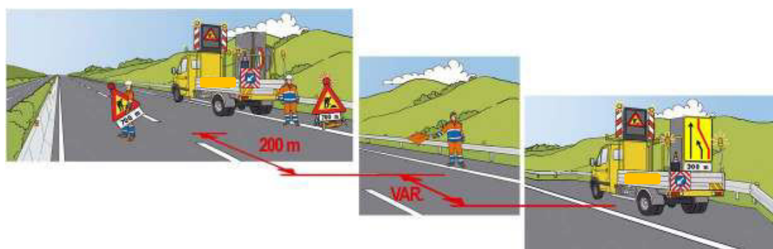
Figura 44 – Chiusura della corsia di marcia: installazione del segnale di lavori in corso sul margine sinistro
