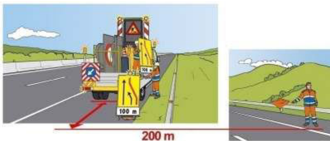
Figura 27 – Chiusura della corsia di marcia: scarico ed installazione sul margine destro dei segnali di riduzione ad una corsia
