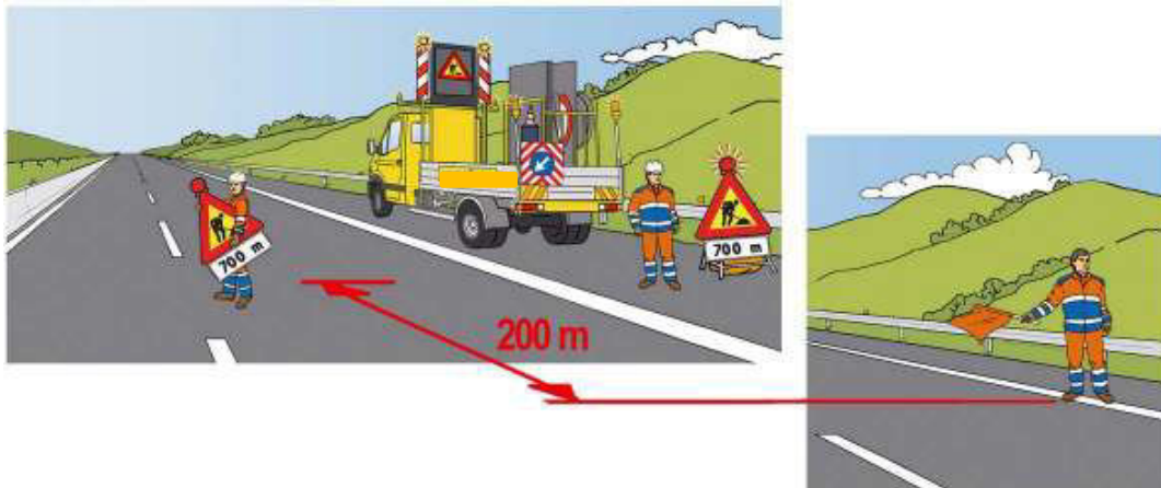
Figura 26 – Chiusura della corsia di marcia: installazione del segnale lavori sul margine sinistro
