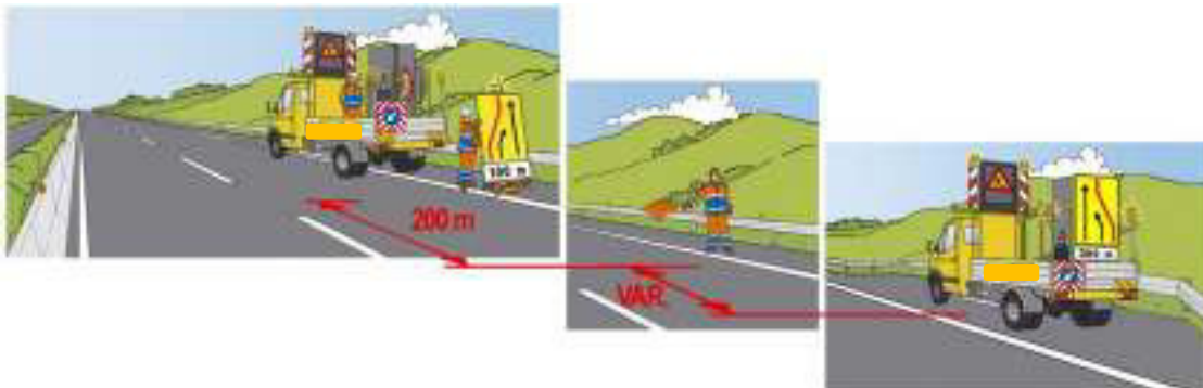
Figura 52 – Chiusura della corsia di sorpasso: installazione del segnale di esclusione della corsia sul margine destro
