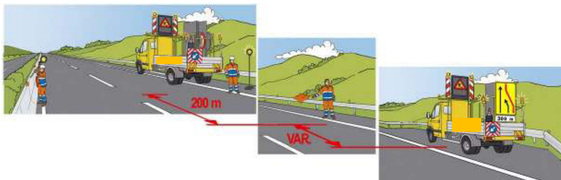
Figura 43 – Chiusura della corsia di marcia: installazione della lampada blitz sul margine sinistro
