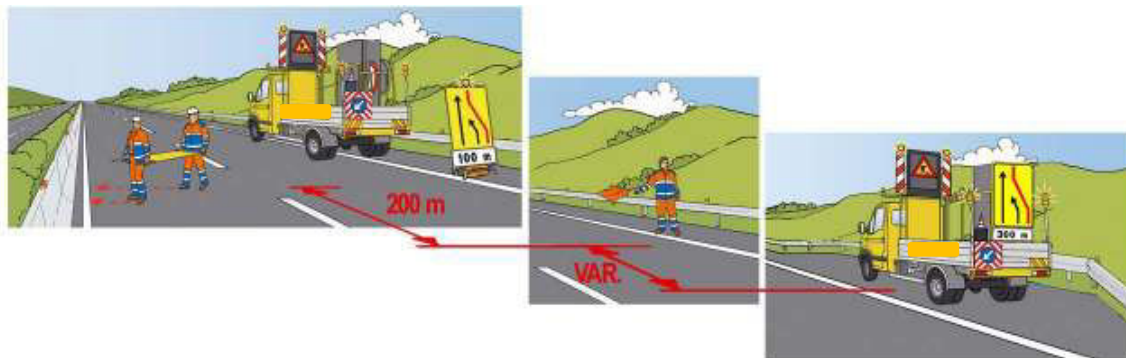
Figura 46 – Chiusura della corsia di marcia: trasporto del segnale di esclusione della corsia sul margine sinistro
