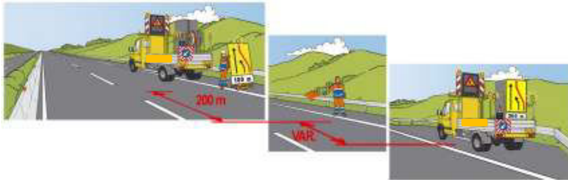
Figura 45 – Chiusura della corsia di marcia: installazione del segnale di esclusione della corsia sul margine destro
