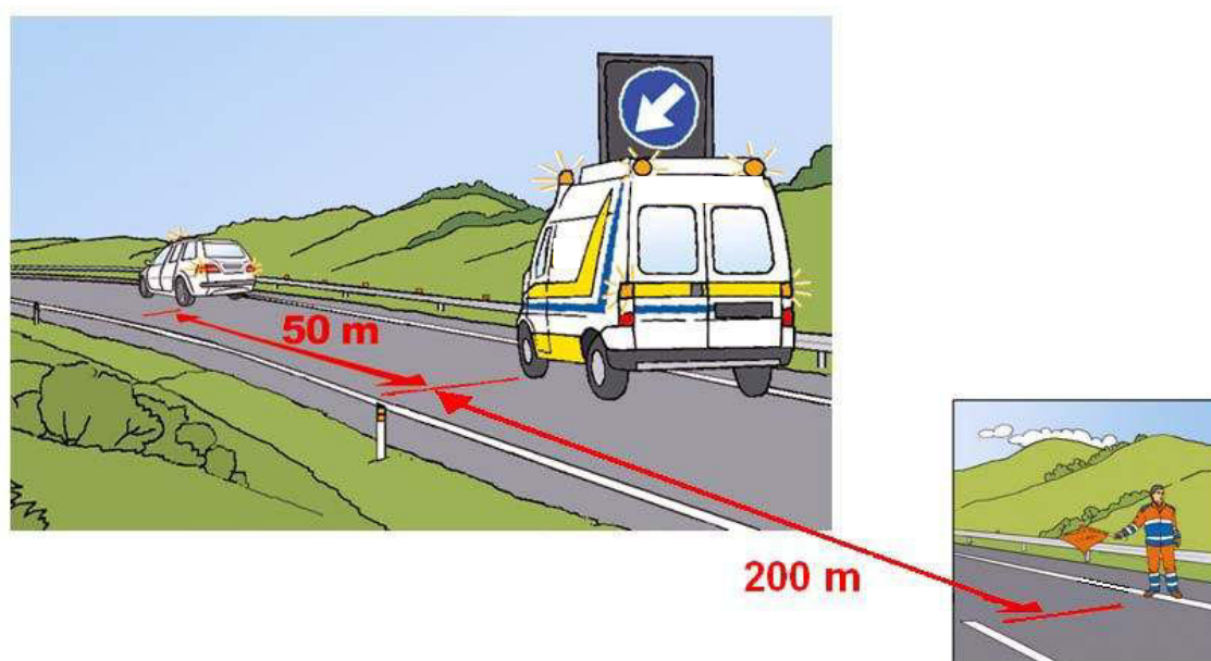
Figura 15 – Fermata del veicolo su tratto senza corsia di emergenza
