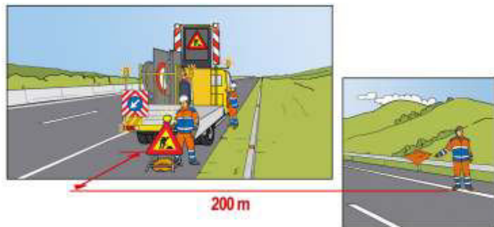
Figura 21 bis – Chiusura della corsia di emergenza: installazione del segnale lavori
