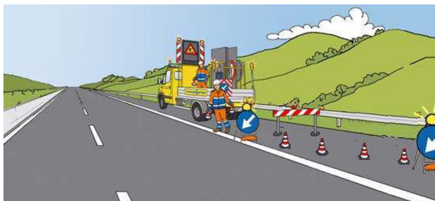
Figura 22 – Chiusura della corsia di emergenza: installazione della testata di chiusura
