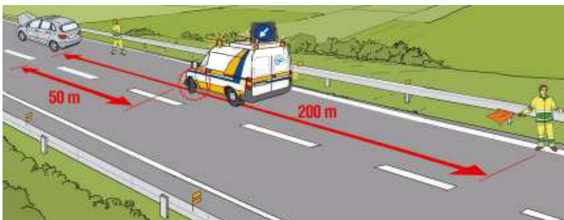
Figura 60 – Fermata del mezzo in tratte di carreggiata prive di corsia di emergenza (esempio corsia di marcia)
