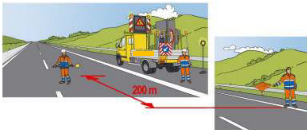
Figura 33 – Chiusura della corsia di sorpasso: installazione della lampada blitz sul margine sinistro
