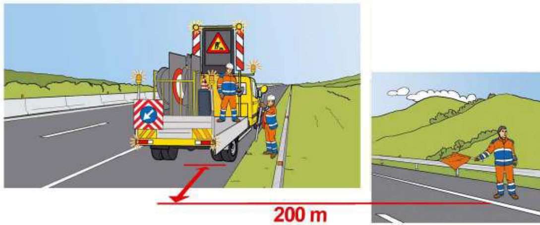
Figura 23 – Chiusura della corsia di marcia: scarico della segnaletica dal mezzo
