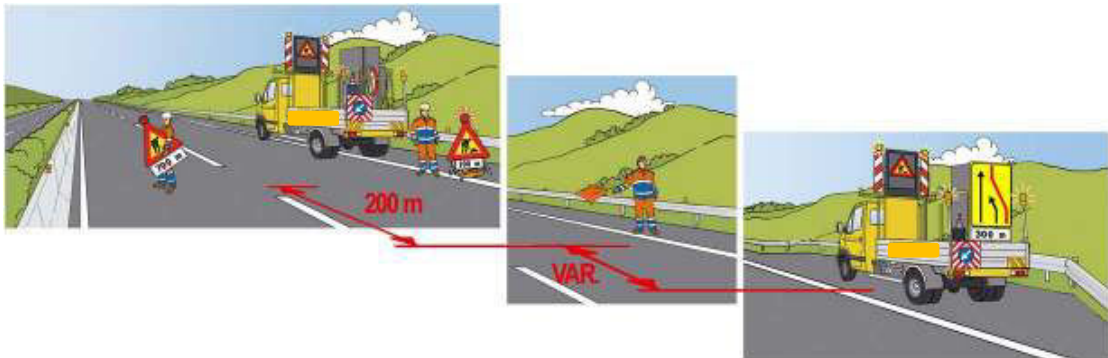
Figura 51 – Chiusura della corsia di sorpasso: installazione del segnale di lavori in corso sul margine sinistro
