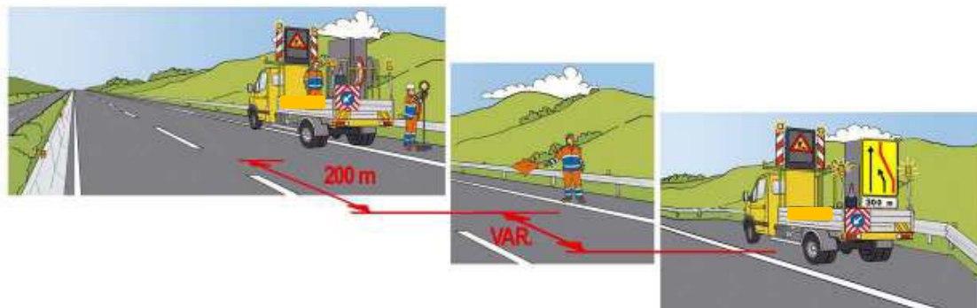
Figura 42 – Chiusura della corsia di marcia: configurazione mezzo di preavviso-sbandiatore-mezzo d'opera
