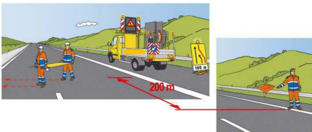
Figura 28 – Chiusura della corsia di marcia: trasporto del segnale di riduzione ad una corsia sul margine sinistro
