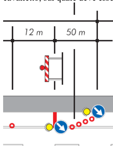
fig. 5 segnaletica di esclusione corsia di emergenza
