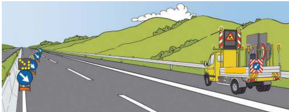
Figura 39 – Chiusura della corsia di sorpasso: installazione della testata di esclusione della corsia
