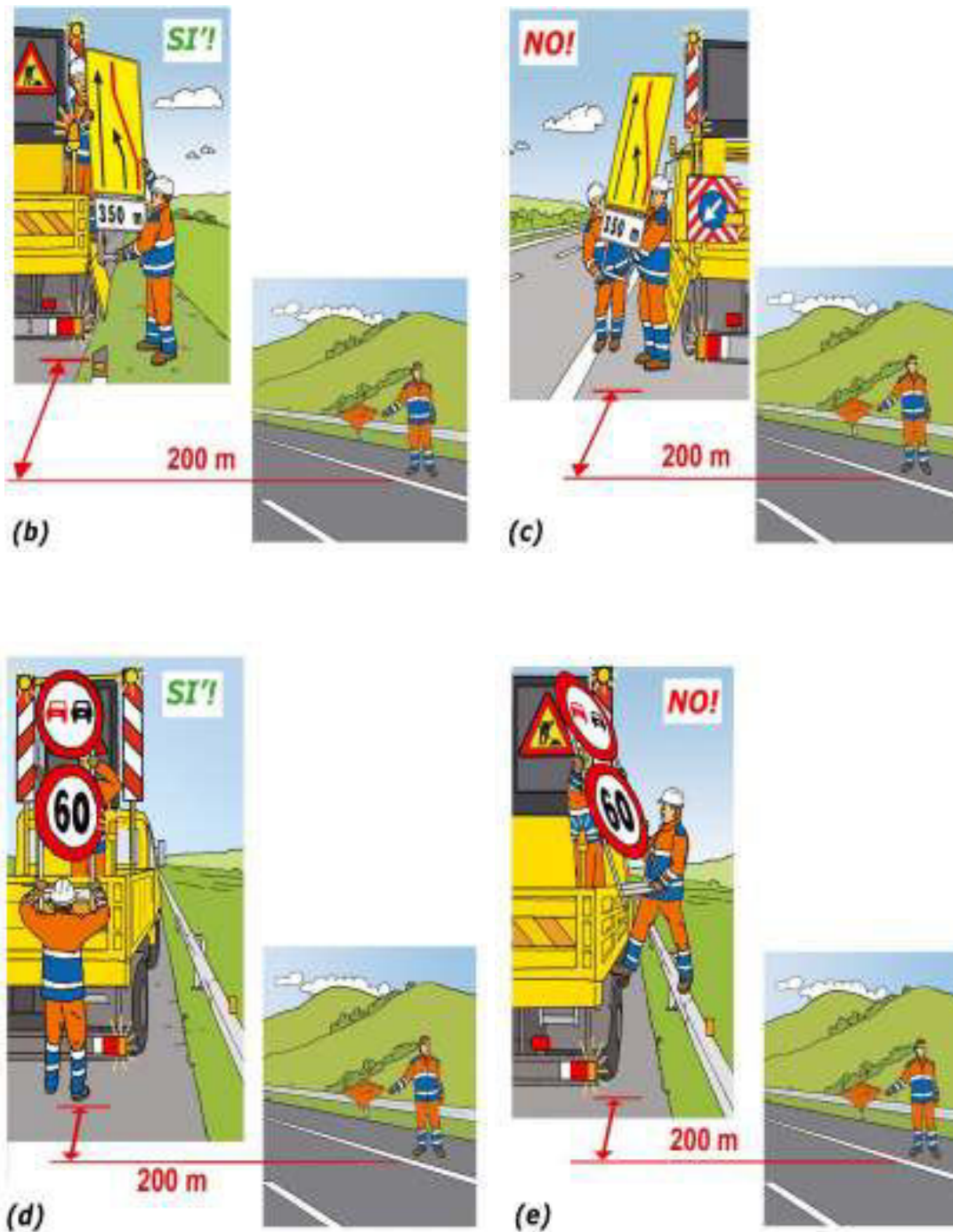
Figura 19 – Prelevamento della segnaletica da automezzo: comportamenti corretti (a), (b), (d) e scorretti (c), (e)
