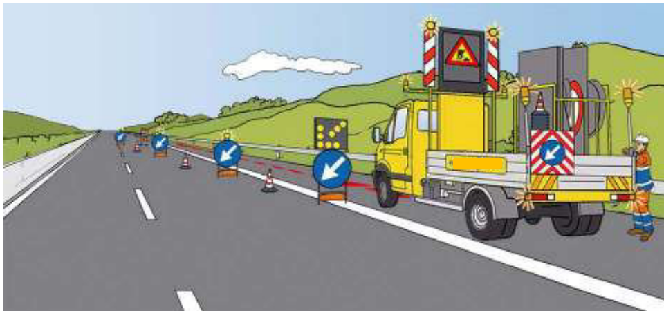
Figura 30 – Chiusura della corsia di marcia: installazione della testata di esclusione della corsia
