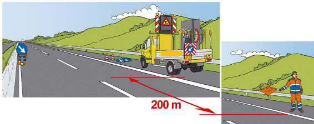
Figura 38 – Chiusura della corsia di sorpasso: inizio installazione della testata di esclusione della corsia
